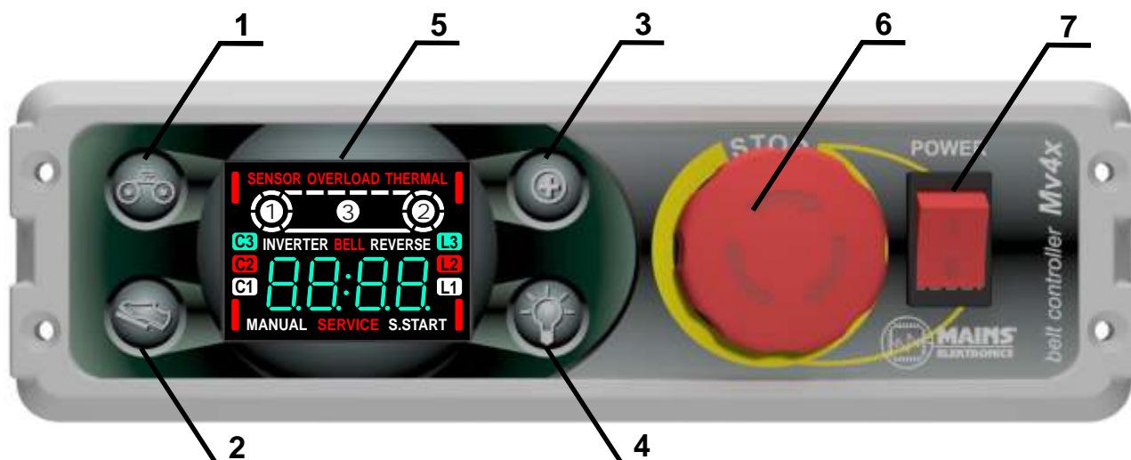
Panel czołowy sterownika MV4X
